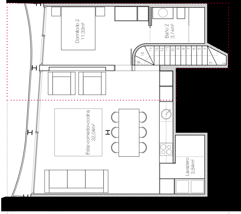
PLANTA PRIMERA
